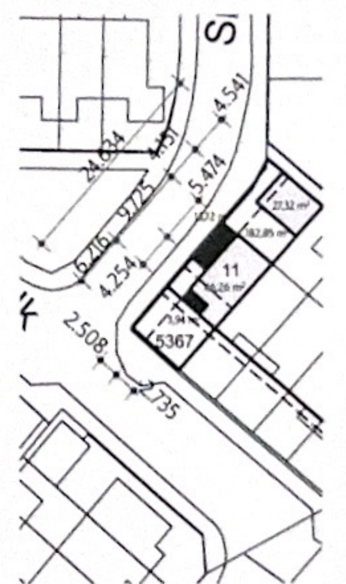
SB SITUATIE
