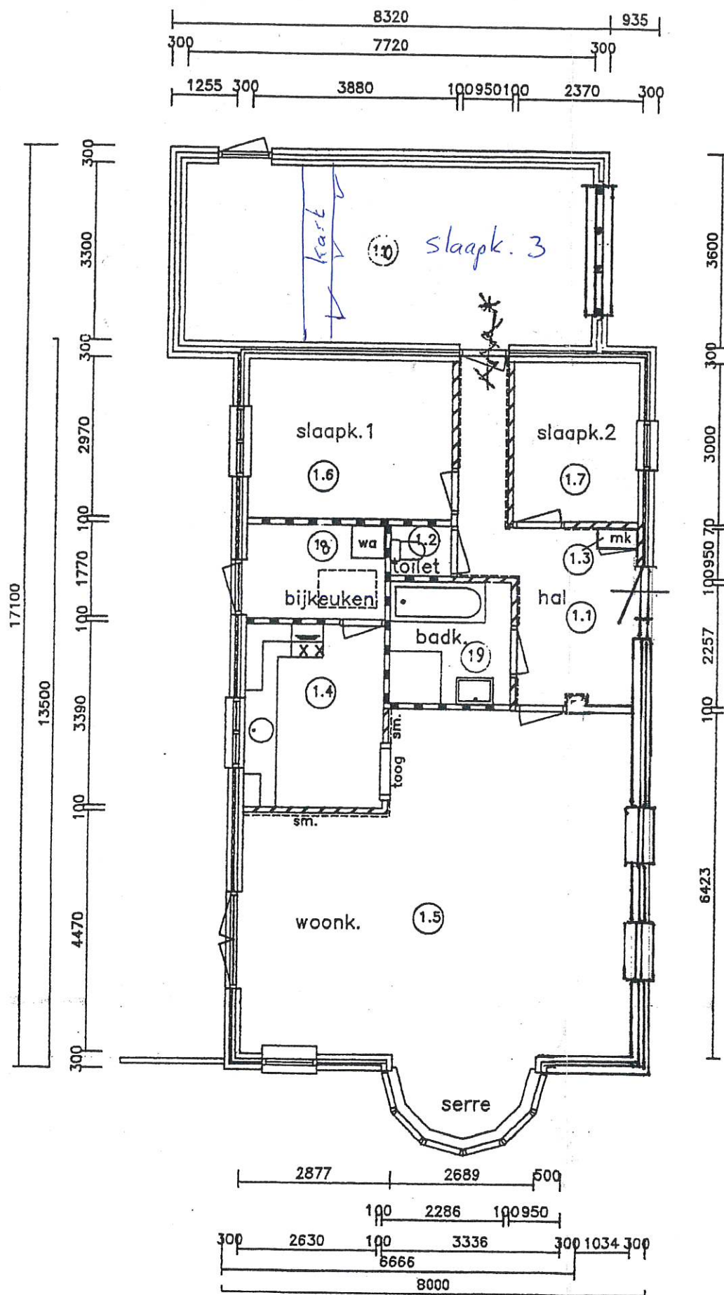
Gewijzigde begane grond
