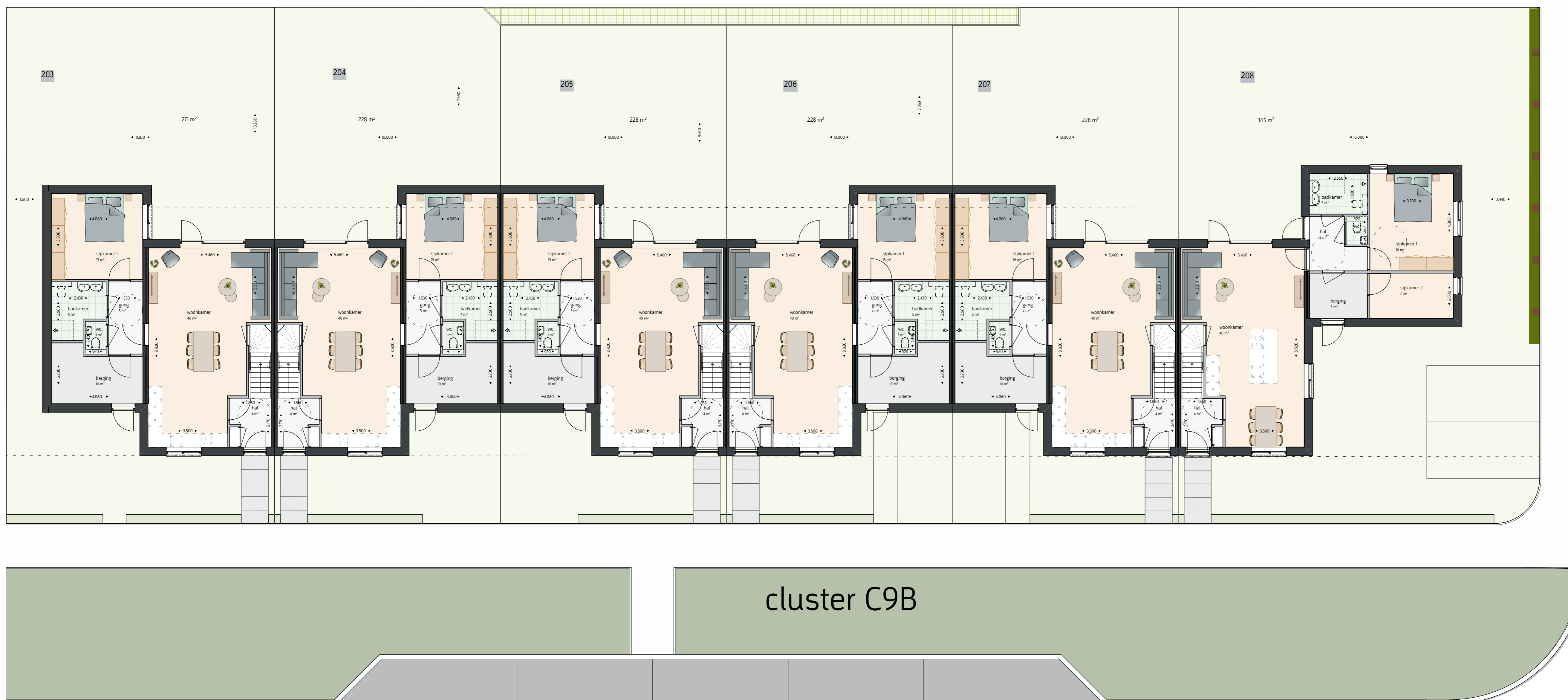
Begane grond
