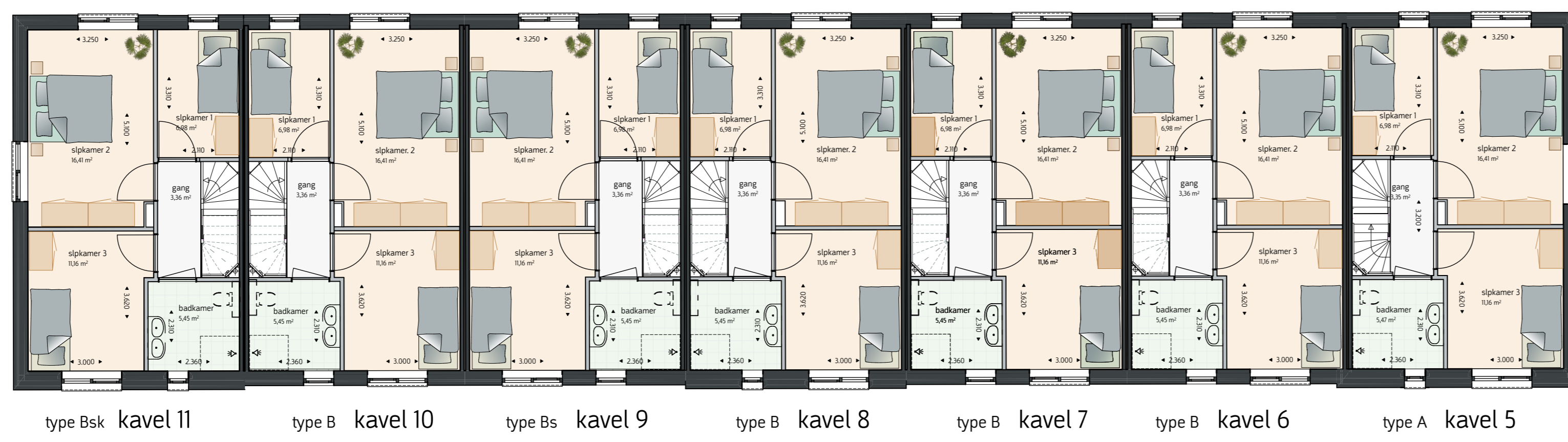
1e verdieping
