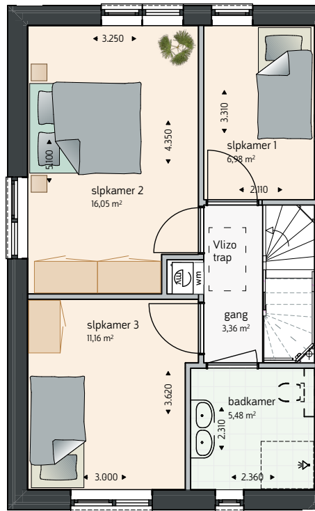
1e verdieping
