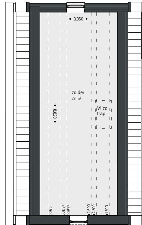
2e verdieping
