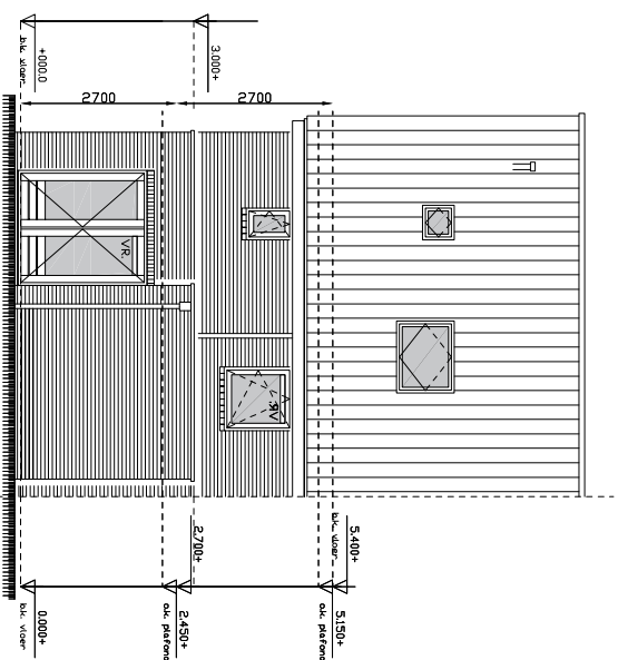
ACHTERGEVEL GEWIJZIGD
